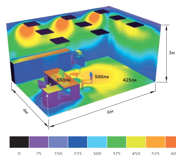
Светодиодные светильники «ОФИС»
