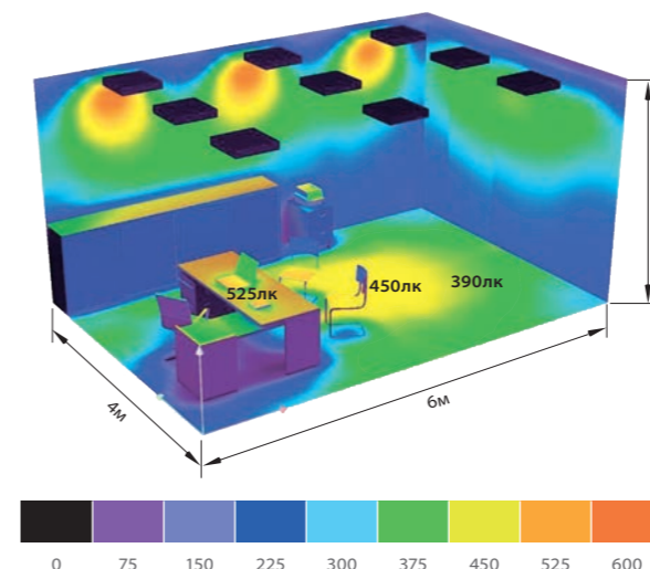
Люминесцентные светильники «ЛВО 4x18»
