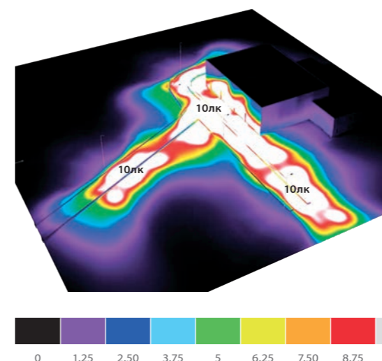
Светильники «PKY 250»
